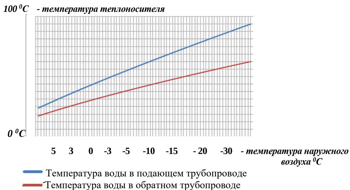
Рис. № 3 - Температурный график качественного регулирования 95/70 °C
